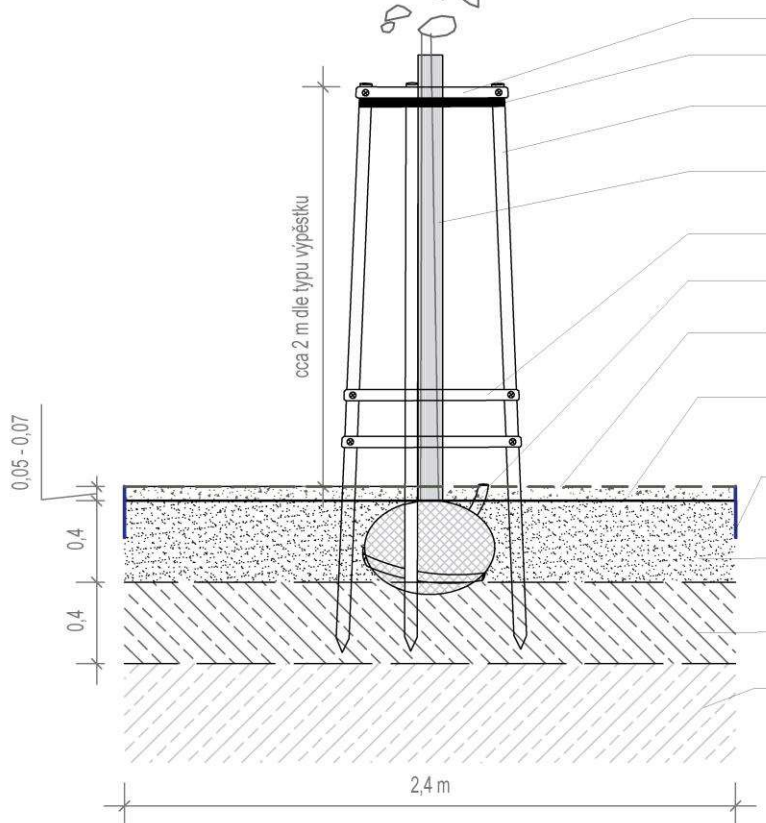
Výsadba stromů – modelový řez
