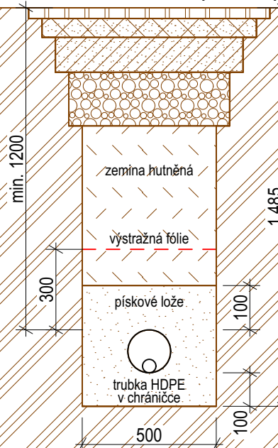
ŘEZ VOZOVKOU (M 1:20)
