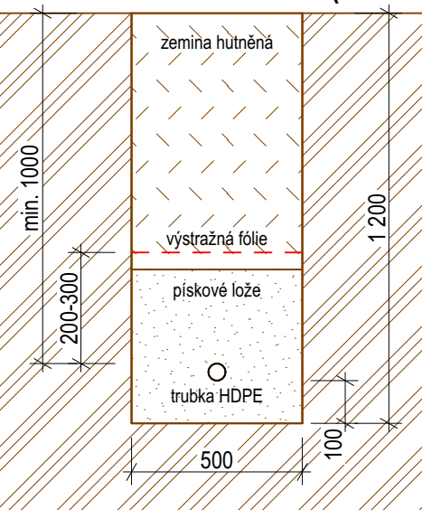
ŘEZ ZELENÝM PRUHEM (M 1:20)
