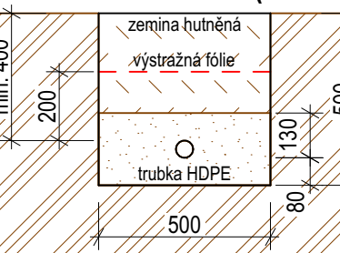
ŘEZ CHODNÍKEM (M 1:20)
